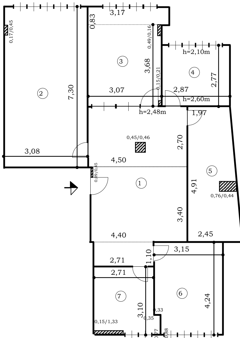
Скица основе канцеларијског простора
